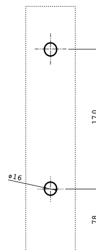
Prumo em tubular quad.40 p/guarda de Vidros
